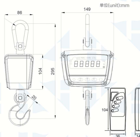
单位(unit):mm
